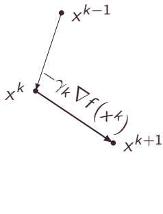
Рис. 3: Градиентный спуск
