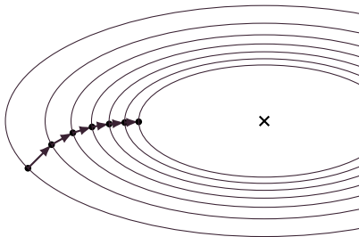
Рис. 1: Градиентный спуск.
